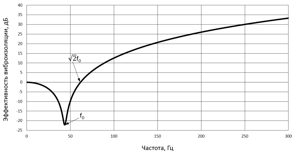
Рисунок 7.1 Эффективность одномассовой виброзащитной системы
