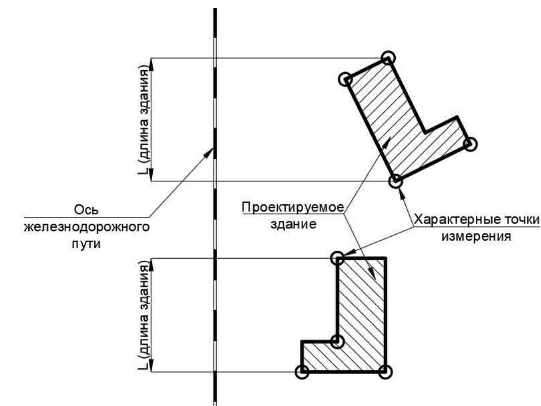
Рисунок Б.2 Рекомендуемые точки измерений в месте расположения здания
