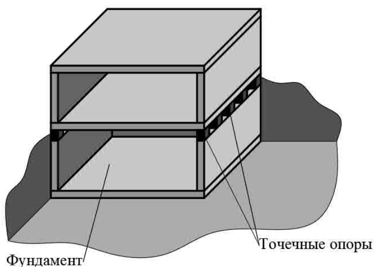
Рисунок 8.1 Схема виброизоляции № 1
