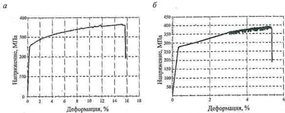
Рисунок К.2 – Обобщенная расчетная диаграмма работы строительных сталей
