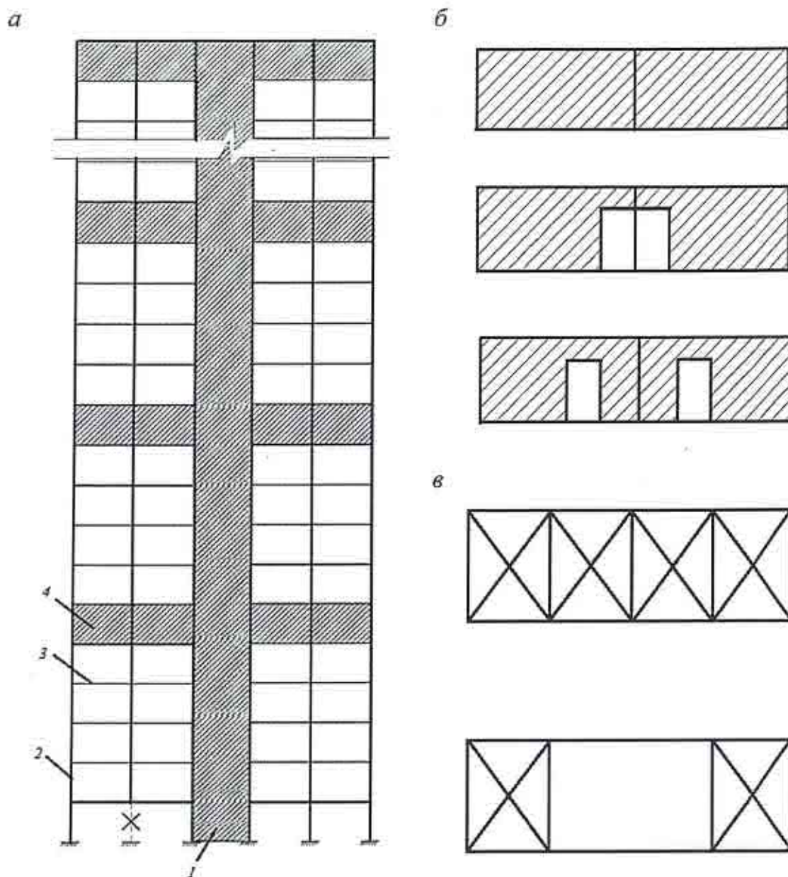
1 – ядро жесткости; 2 – колонны; 3 – ригели; 4 – аутриггерная конструкция
