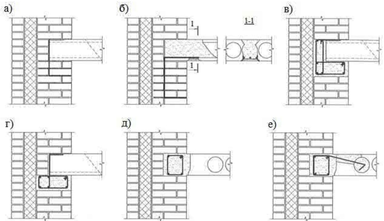
Рисунок Ж.4 – Варианты укладки дополнительной арматуры с увеличенным защитным слоем в монолитных участках при монтаже (а), плитах перекрытия при изготовлении (б) и замоноличенных пустотах плит перекрытия (в)
