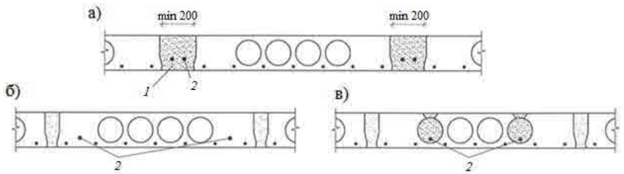
Рисунок Ж.4 – Варианты укладки дополнительной арматуры с увеличенным защитным слоем в монолитных участках при монтаже (а), плитах перекрытия при изготовлении (б) и замоноличенных пустотах плит перекрытия (в)
