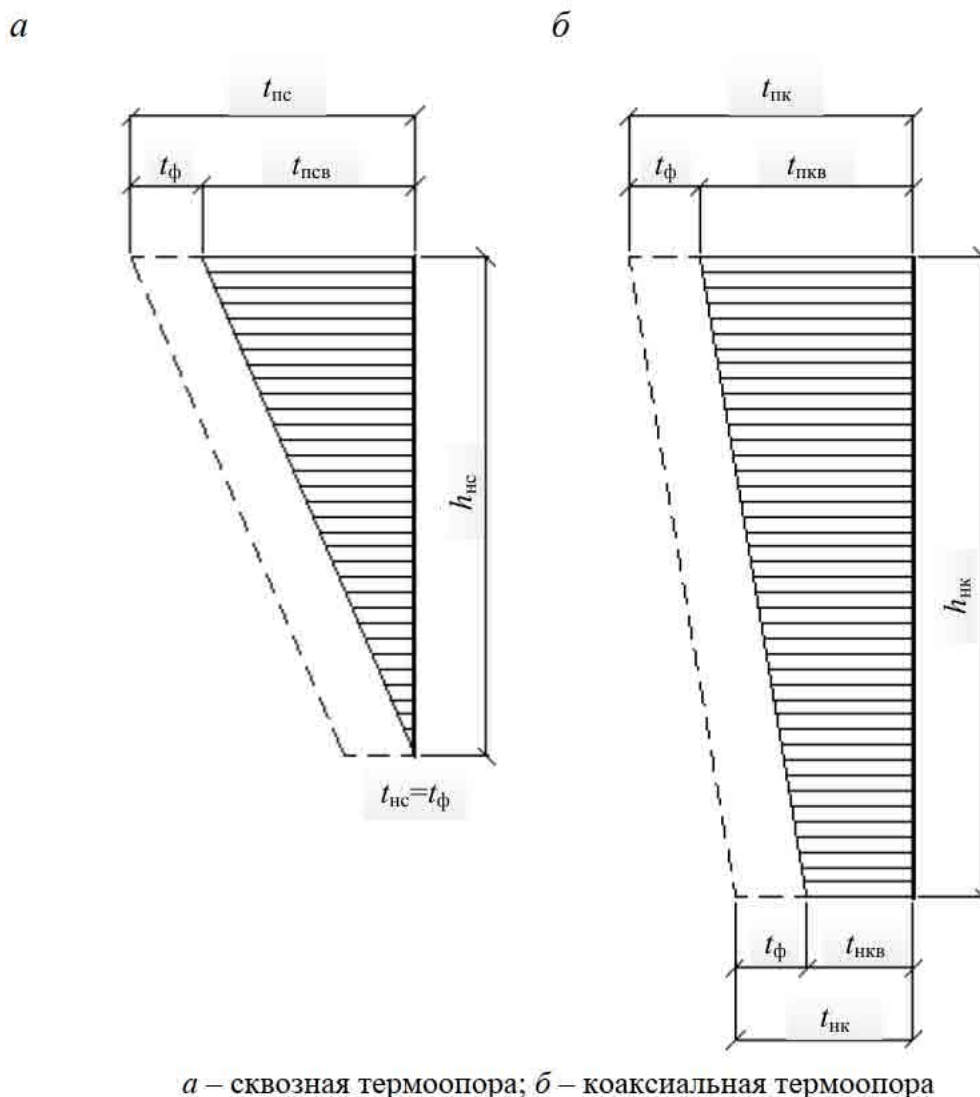
Рисунок И.3 Расчетные эпюры температур воздуха в полости сквозной и коаксиальной термоопор
