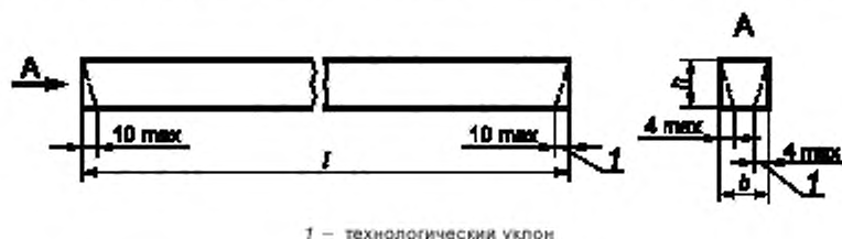
Рисунок 1 — Перемычка типа ПБ
