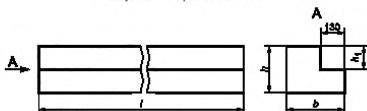
Рисунок 3 — Перемычка типа ПГ
