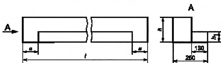
Рисунок 4 — Перемычка типа ПФ
