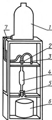
1 — склянка 3—3 по ГОСТ 25336—82; 2, 5 — краны; 3, 7 — резиновые трубки; 4 — бюретка; 6 — сосуд
