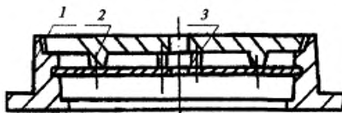
Рисунок А.2 — Люк, оснащенный запорным замковым устройством
