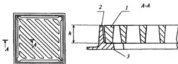
Рисунок Б.1 — Дождеприемник ливнесточного колодца
