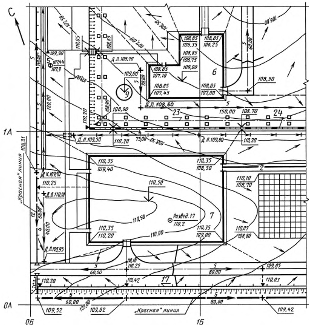
Пример оформления плана организации рельефа в проектных отметках
