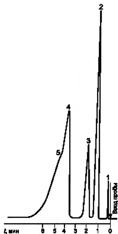
Типовая хроматограмма растворителя марки 647
