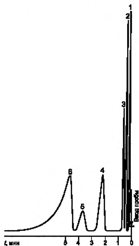
Типовая хроматограмма растворителя марки 646
