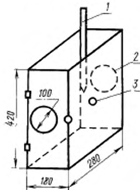
1 — пипетка; 2 — смотровое стекло; 3 — отверстие для зажима
