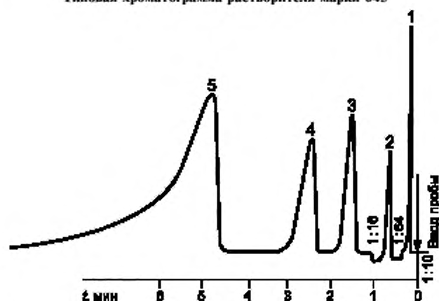
Типовая хроматограмма растворителя марки 645
