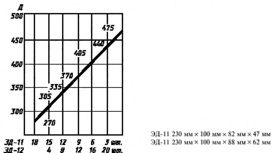
Рисунок В.1 — Свод толщиной 230 мм
