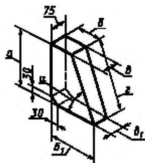
Рисунок 8 — Опорный кирпич
