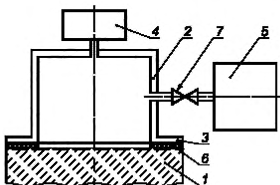
1 — бетонный образец; 2 — камера устройства; 3 — фланец камеры; 4 — вакуумметрический датчик; 5 — вакуумноса; 6 — герметизирующая мастика; 7 — вентиль
